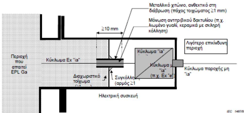
Σχήμα 1 – Παράδειγμα διαχωριστικού τοιχώματος με αντιτριβικό δακτύλιο αγωγών που θεωρείται ότι είναι αεράστεγες
